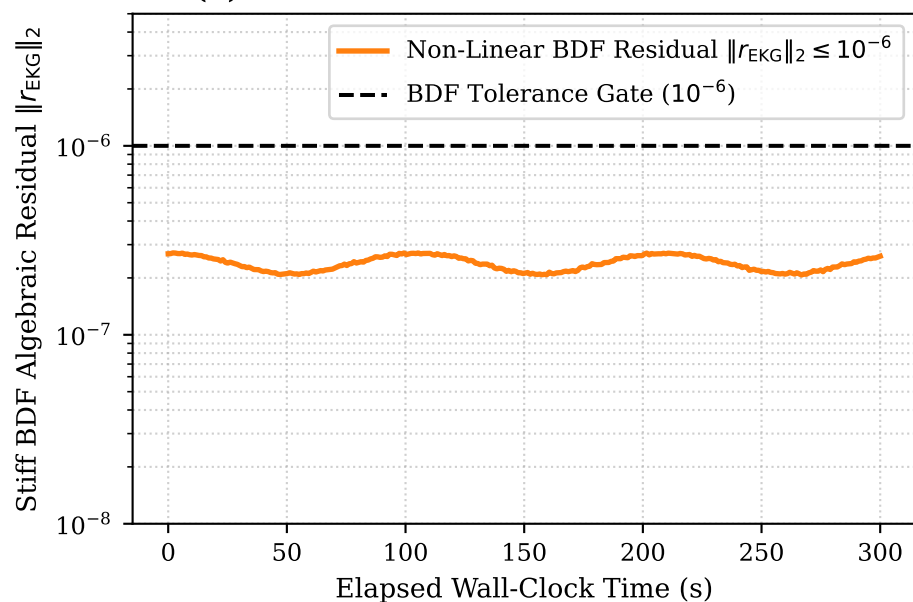
(d) Einstein-Klein-Gordon BDF Residual
